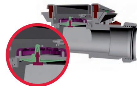
Válvula de aireación cerrada.
