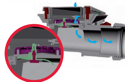
Válvula de aireación abierta.
